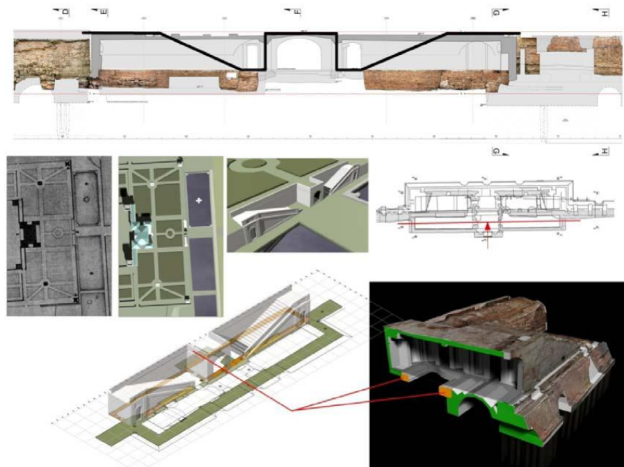
Muzeum Pałac w Wilanowie. Rekonstrukcja grotty i schodów ukazanych na planie Boy'a (1682 r.) w oparciu o zachowane relikty fundamentów.
